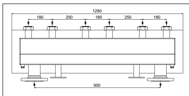
„HydroFixx“ Ду40/50, на 3 отвода
