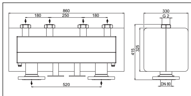
„HydroFixx“ Ду 40/50, на 2 отвода
